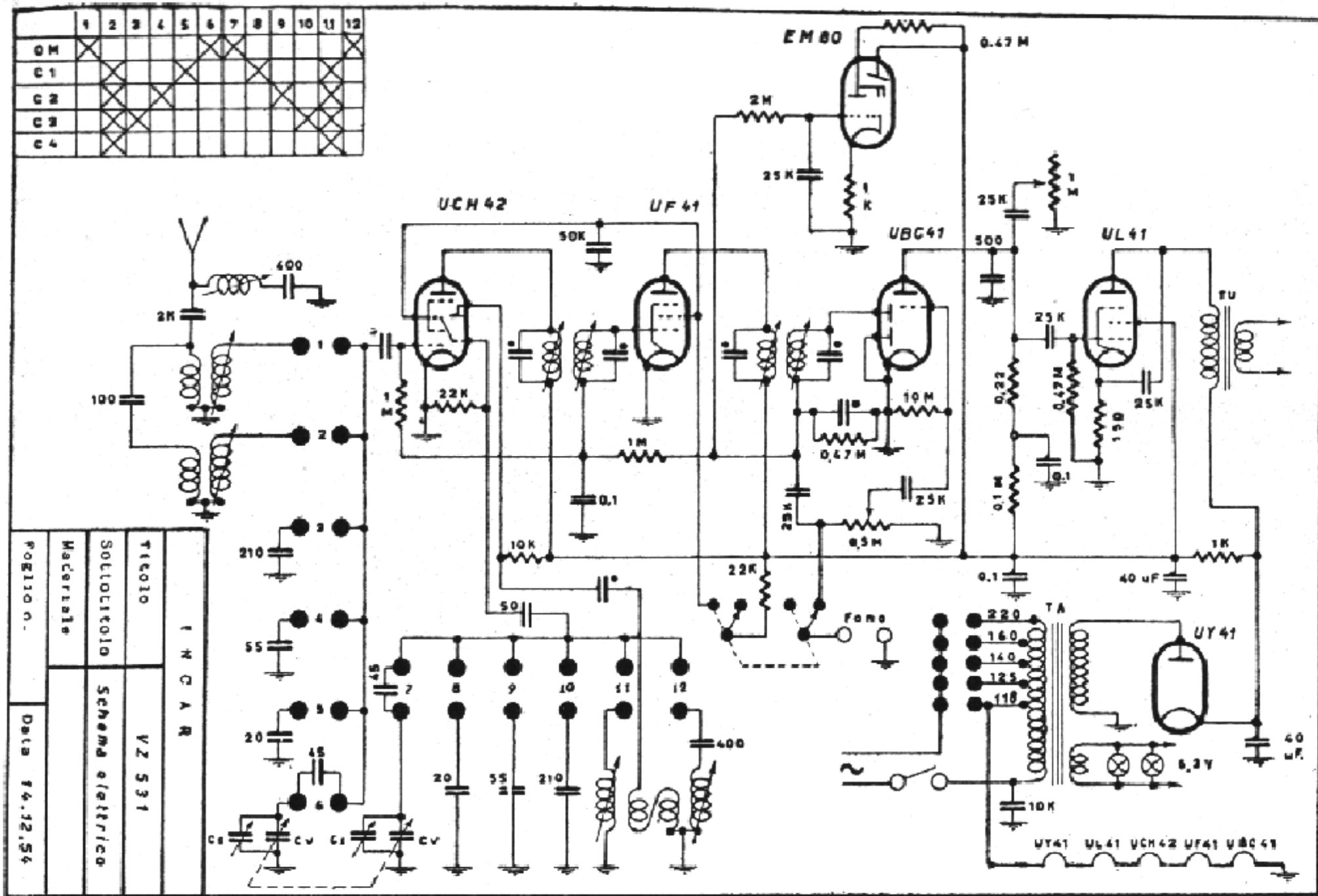
INCAR - Mod. VZ 531 - Ricevitore a onde medie con quattro bande allargate a onde corte. Potenza d'uscita 3 watt. Cons. 50 watt.
